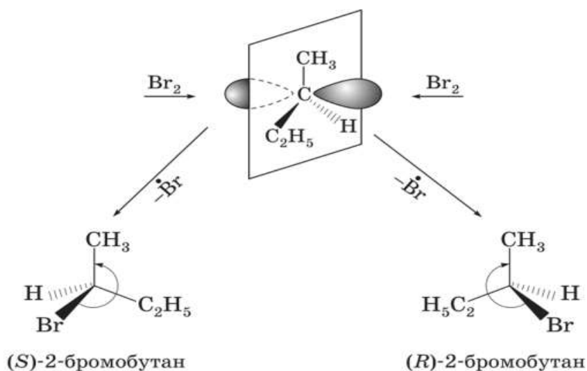
Сурет 2. S_R реакциясының стереохимиясы
