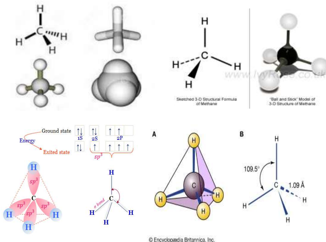
Сурет 3. Метанның 3D құрылысы
