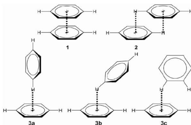
Сурет 1 Бензолдың стереохимиясы
