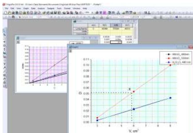
2- сурет. Перманганат пен дихроматтың стандартты ерітінділерінің оптикалық тығыздығын өлшеу нәтижелері бойынша градуирлеу графиктері б) Градуирлеу графиктерінің әдісі
