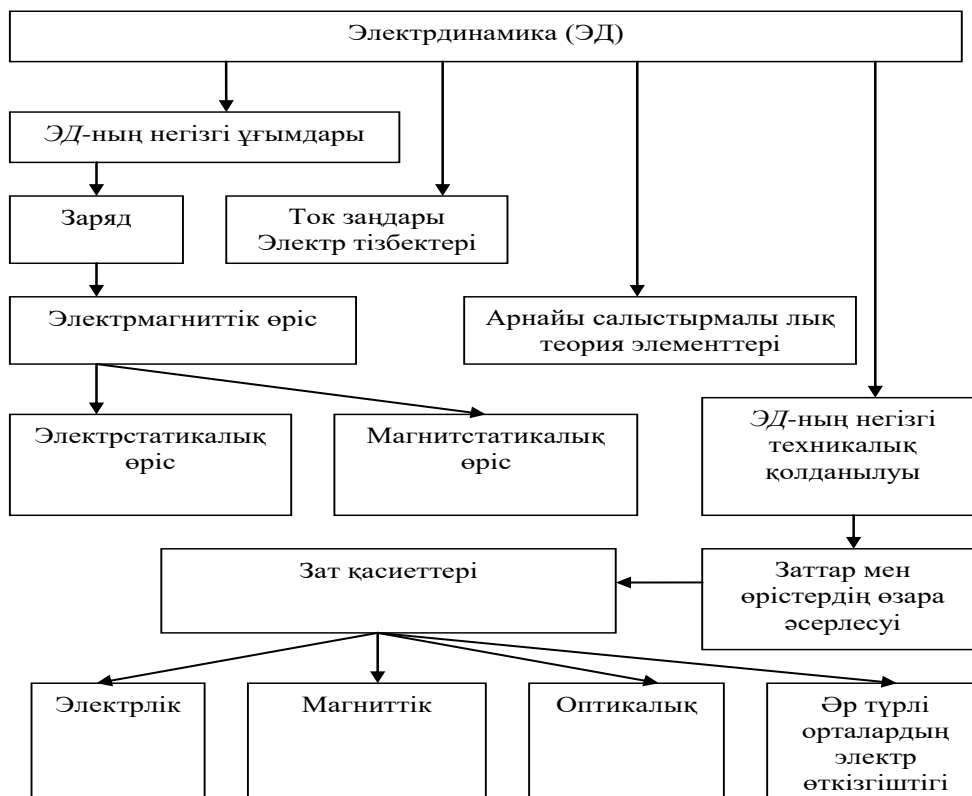
1-кесте. Электродинамика
